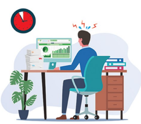
Without DataDora
